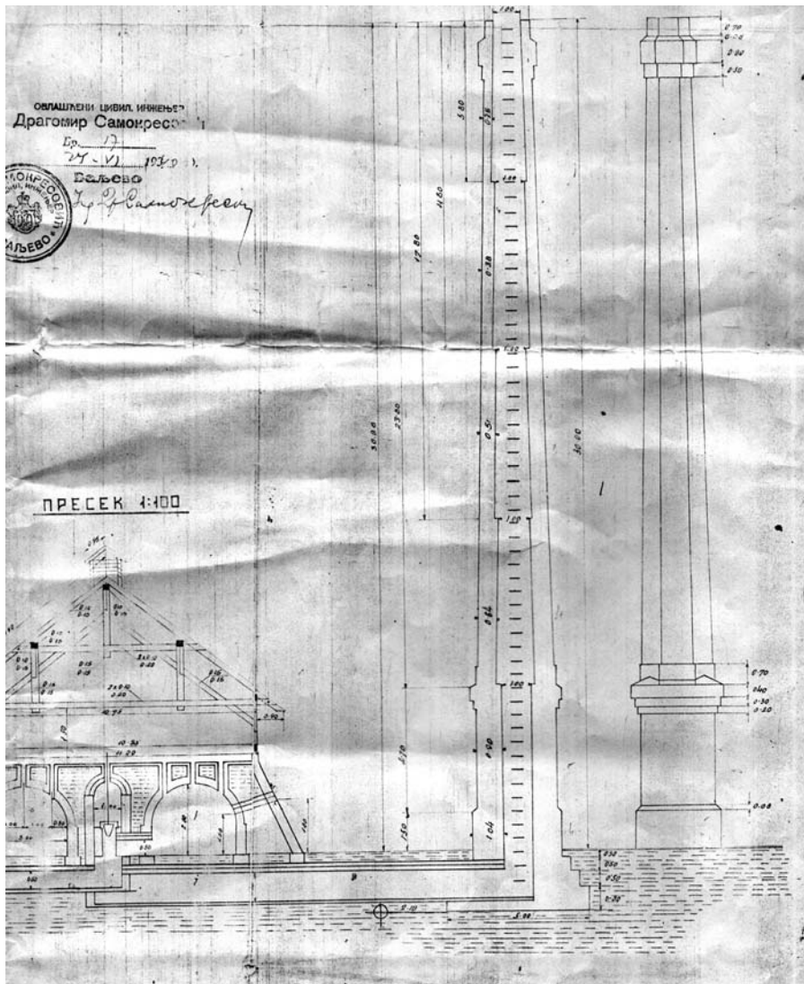
Детаљ пројекта циглане, 1940. године
